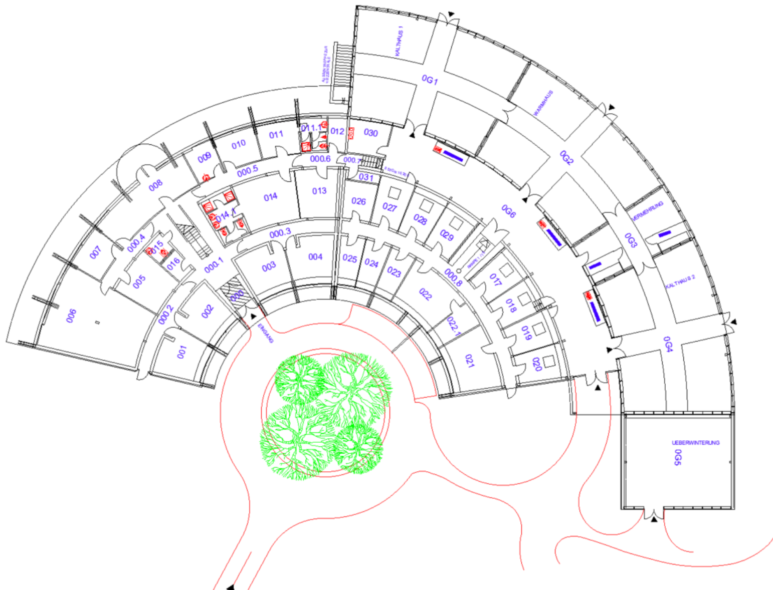
Abbildung 4: Grundriss - Erdgeschoss
