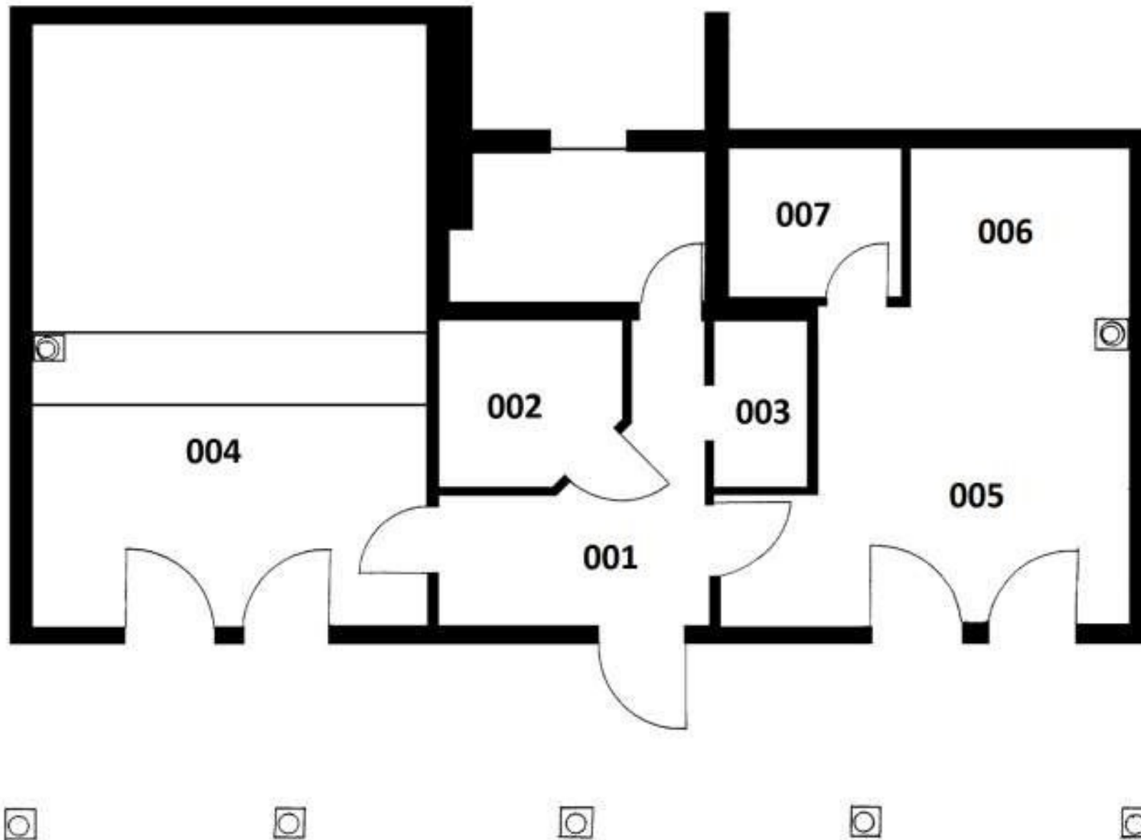
Abbildung 15: Grundriss - Erdgeschoss
