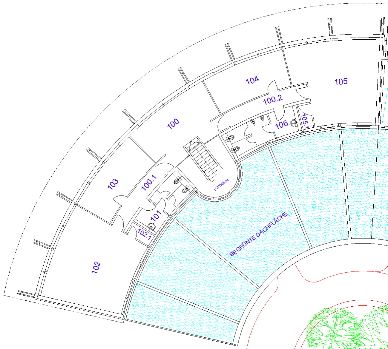
Abbildung 5: Grundriss - Erste Etage
